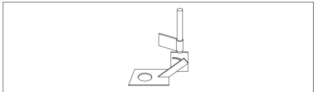
图 23 通用安装支座（1.4301 材质），配备倾转装置和固定头，传感器开孔直径 \varnothing 108 mm (4.25 in)
