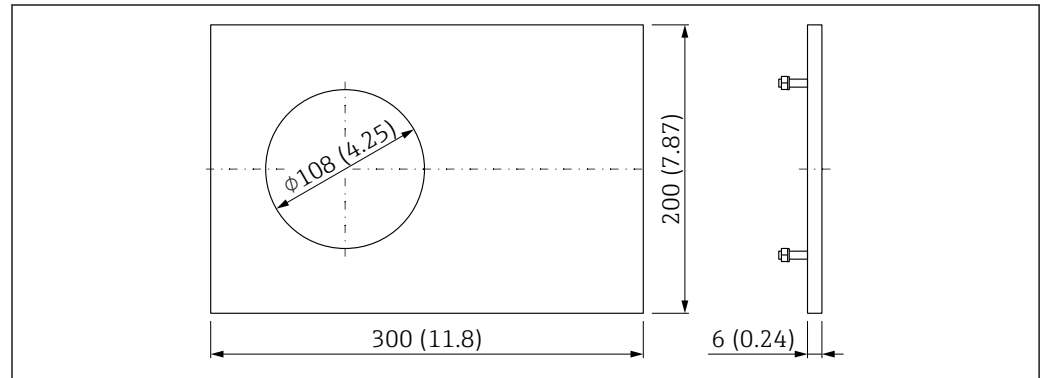
图 22 挡板，1.4301，传感器开孔 \varnothing 108 mm (4.25 in)。测量单位 mm (in)
