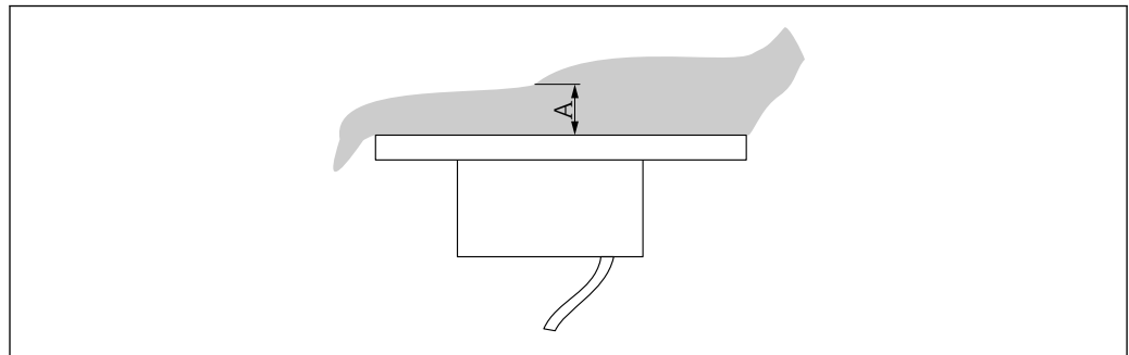
图 27 传感器顶部的物料高度
